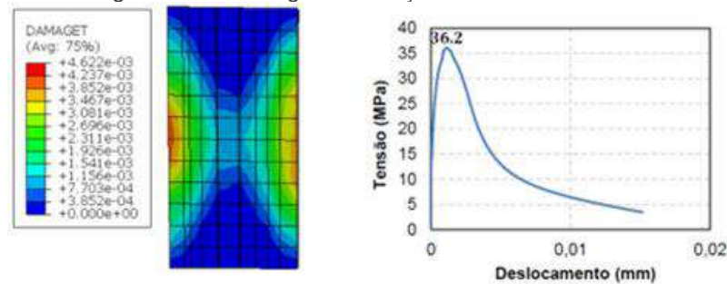
Figura 12. Modelagem no traço 2% de fibra hooked
