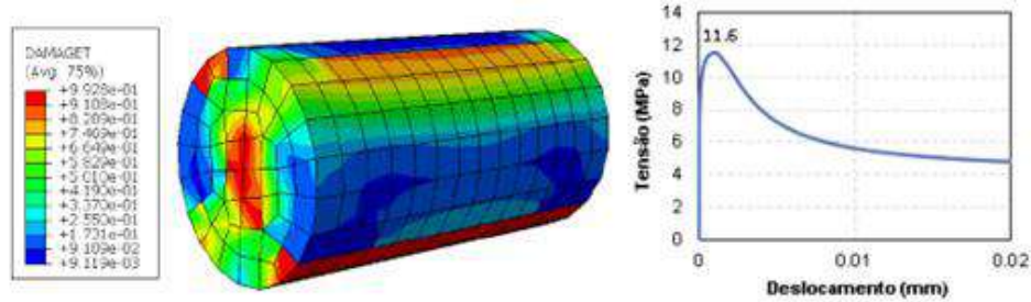
Figura 15. Modelagem do corpo de prova com 2% de Fibra Crimped (CD2%)
