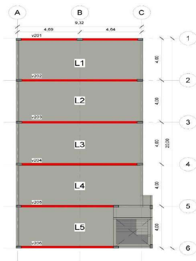
Figura 3. Planta do pavimento superior
