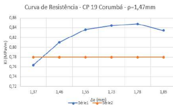
Figura 4. Curva de Resistencia – CP19 - Cinza Corumbá \rho=1,47\text{mm}
